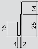
Рис. 6.2. Кутник зовнішній
