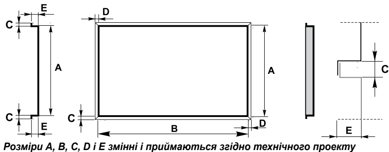
Рис. 9. Касетон T-1
